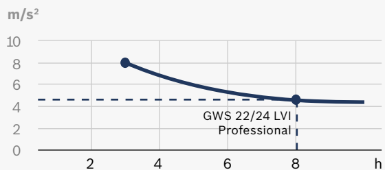
Vibrațiile sculei electrice în m/s^2
